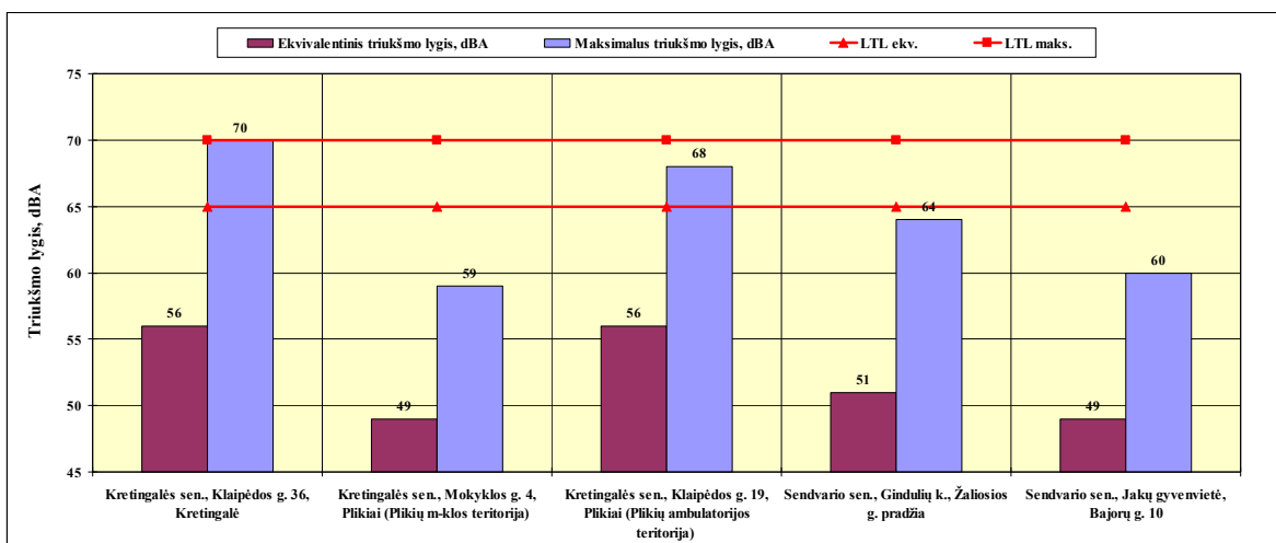
4.9 pav. Ekvivalentiniai ir maksimalūs triukšmo lygiai nustatyti rytinio piko metu Kretingalės, Sendvario ir Judrėnų seniūnijose
