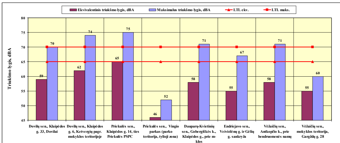
4.8 pav. Ekvivalentiniai ir maksimalūs triukšmo lygiai nustatyti rytinio piko metu Dovilų, Priekulės, Dauparų-Kvietinių, Endriejavo ir Vėžaičių seniūnijose
