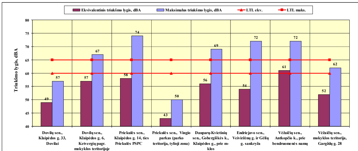
4.11 pav. Ekvivalentiniai ir maksimalūs triukšmo lygiai nustatyti rytinio piko metu Dovių, Priekulės, Dauparų-Kvietinių, Endriejavo ir Vėžaičių seniūnijose
