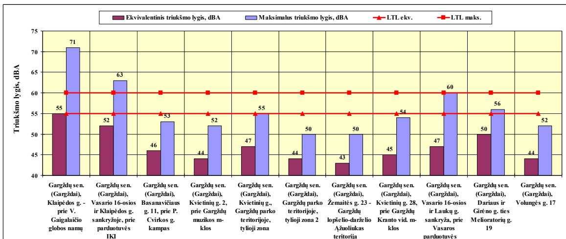
4.13 pav. Ekvivalentiniai ir maksimalūs triukšmo lygiai nustatyti nakties metu Gargždų mieste
