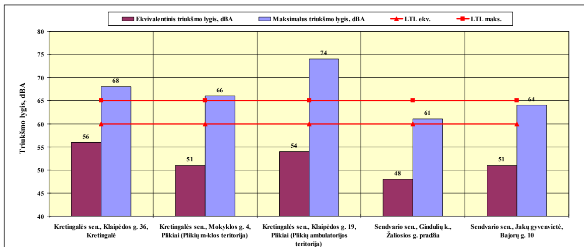
4.12 pav. Ekvivalentiniai ir maksimalūs triukšmo lygiai nustatyti vakarinio piko metu Kretingalės, Sendvario ir Judrėnų seniūnijose
