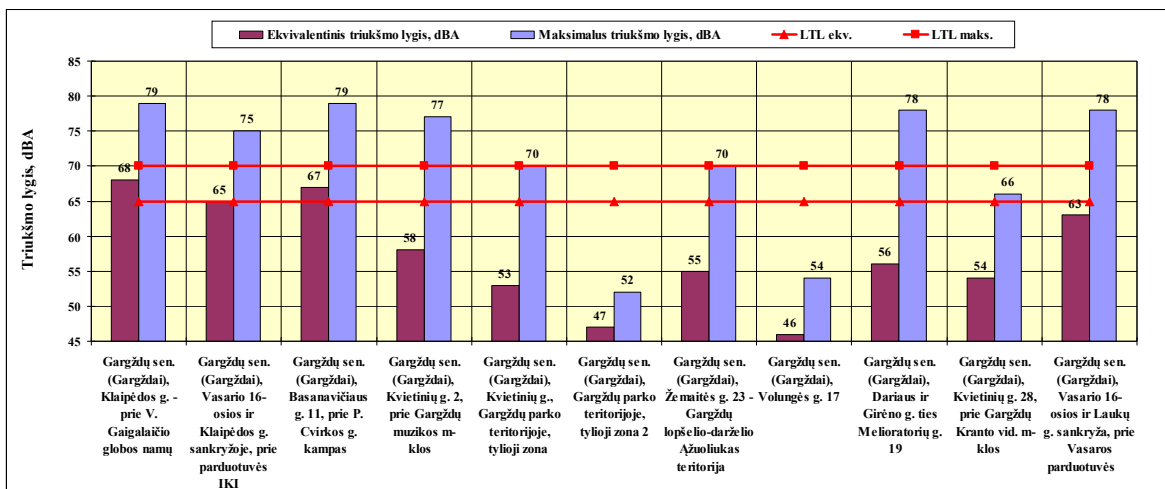
4.7 pav. Ekvivalentiniai ir maksimalūs triukšmo lygiai nustatyti rytinio piko metu Gargždų mieste
