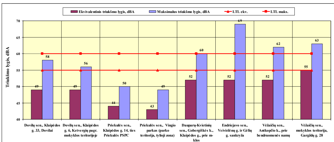
4.14 pav. Ekvivalentiniai ir maksimalūs triukšmo lygiai nustatyti nakties metu Dovylių, Priekulės, Dauparų-Kvietinių, Endrijevavo ir Vėžaičių seniūnijose
