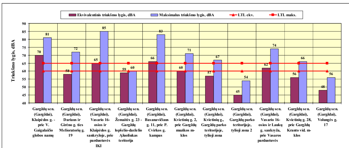
4.10 pav. Ekvivalentiniai ir maksimalūs triukšmo lygiai nustatyti vakarinio piko metu Gargždų mieste
