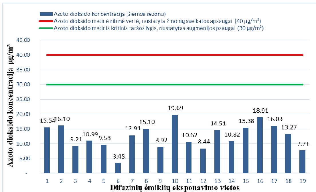
2.1 pav. Azoto dioksido (NO 2 ) koncentracija aplinkos ore Klaipėdos rajone 2018 m. žiemos sezono metu bei metinė ribinė vertė, nustatyta žmonių sveikatos apsaugai (40 µg/m 3 ) ir metinis kritinis taršos lygis, nustatytas augmenijos apsaugai (30 µg/m 3 )
