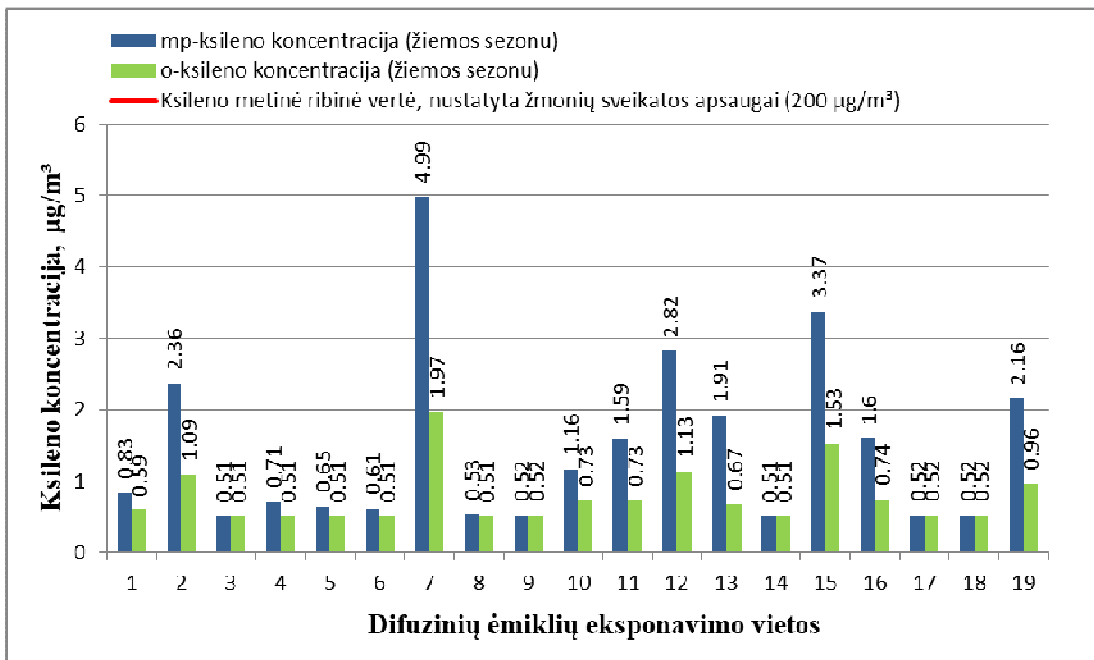
2.6 pav. m/p-ksileno ir o-ksileno paros koncentracija aplinkos ore Klaipėdos rajone 2018 m. žiemos sezono metu (ksileno paros ribinė vertė, nustatyta žmonių sveikatos apsaugai 200 µg/m 3 ) (raudonai pažymėtos reikšmės – žemiau metodo nustatymo ribos)
