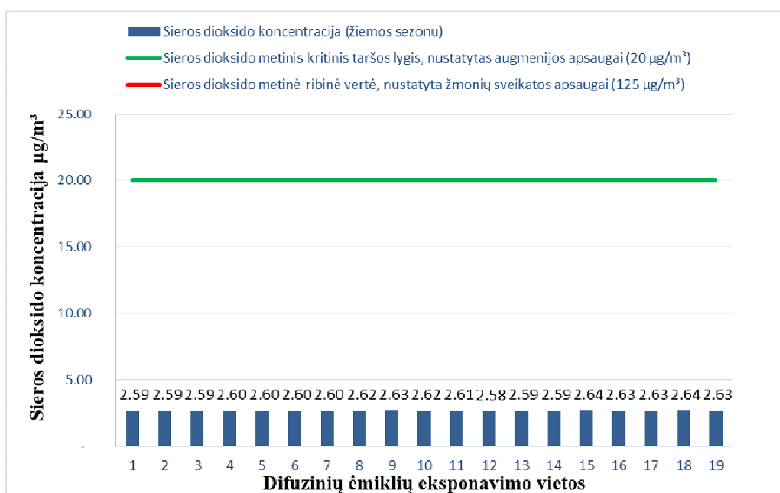
2.2 pav. Sieros dioksido ( \text{SO}_2 ) koncentracija aplinkos ore Klaipėdos rajone 2018 m. žiemos sezono metu (paros ribinė vertė, nustatyta žmonių sveikatos apsaugai ( 125 \mu\text{g}/\text{m}^3 ) ir metinis kritinis taršos lygis, nustatytas augmenijos apsaugai ( 20 \mu\text{g}/\text{m}^3 )) (raudonai pažymėtos reikšmės – žemiau metodo nustatymo ribos)
