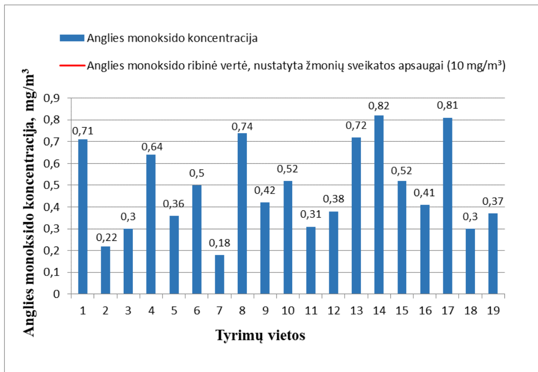
2.8 pav. Anglies monoksido (CO) koncentracija aplinkos ore Klaipėdos rajone 2018 m. žiemos sezono metu bei ribinė vertė, nustatyta žmonių sveikatos apsaugai (10 mg/m 3 )
