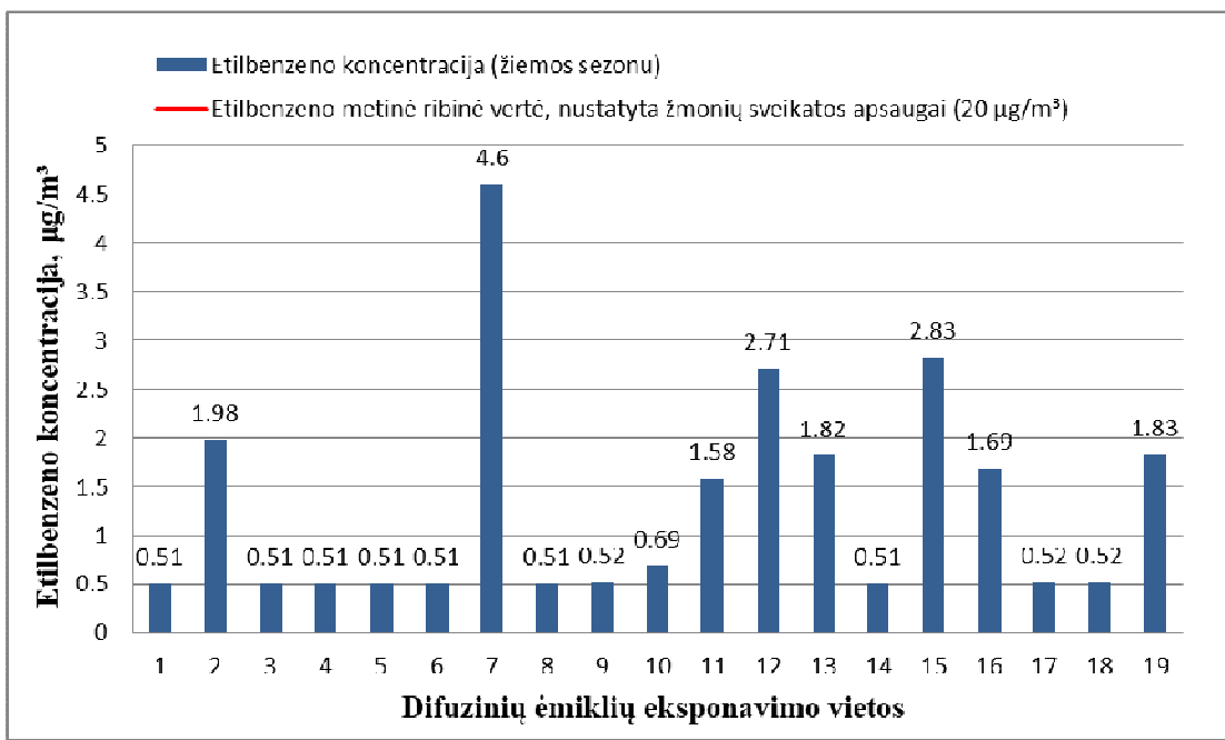
2.5 pav. Etilbenzeno paros koncentracija aplinkos ore Klaipėdos rajone 2018 m. žiemos sezono metu (etilbenzeno paros ribinė vertė, nustatyta žmonių sveikatos apsaugai 20 \mu\text{g}/\text{m}^3 ) (raudonai pažymėtos reikšmės – žemiau metodo nustatymo ribos)
