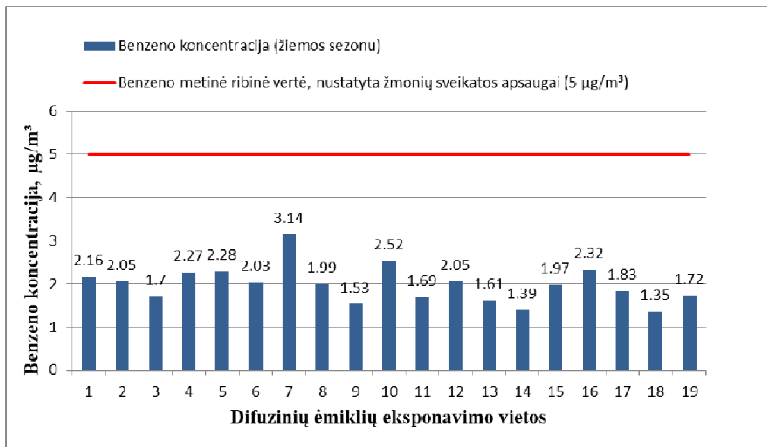
2.3 pav. Benzeno koncentracija aplinkos ore Klaipėdos rajone 2018 m. žiemos sezono metu (benzeno paros ribinė vertė, nustatyta žmonių sveikatos apsaugai 5 \mu\text{g}/\text{m}^3 )
