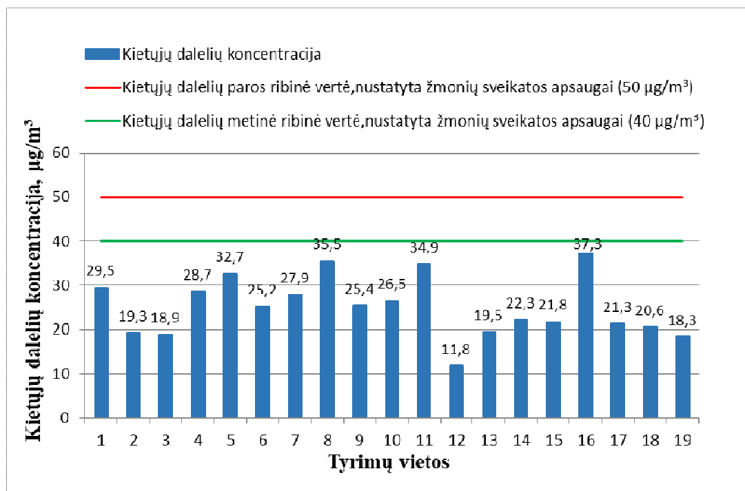
2.7 pav. Kietųjų dalelių (KD 10 ) koncentracija aplinkos ore Klaipėdos rajone 2018 m. žiemos sezono metu bei paros ribinė vertė, nustatyta žmonių sveikatos apsaugai (50 µg/m 3 ) ir metinė ribinė vertė, nustatyta žmonių sveikatos apsaugai (40 µg/m 3 )
