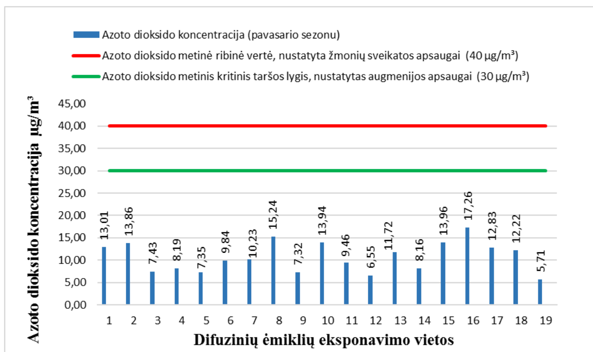
2.1 pav. Azoto dioksido (NO 2 ) koncentracija aplinkos ore Klaipėdos rajone 2020 m. pavasario sezono metu bei metinė ribinė vertė, nustatyta žmonių sveikatos apsaugai (40 µg/m 3 ) ir metinis kritinis taršos lygis, nustatytas augmenijos apsaugai (30 µg/m 3 )
