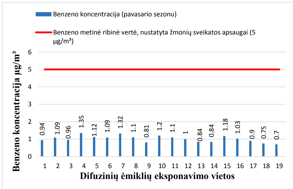
2.3 pav. Benzeno koncentracija aplinkos ore Klaipėdos rajone 2020 m. pavasario sezono metu bei benzene paros ribinė vertė, nustatyta žmonių sveikatos apsaugai ( 5 \mu\text{g}/\text{m}^3 )
