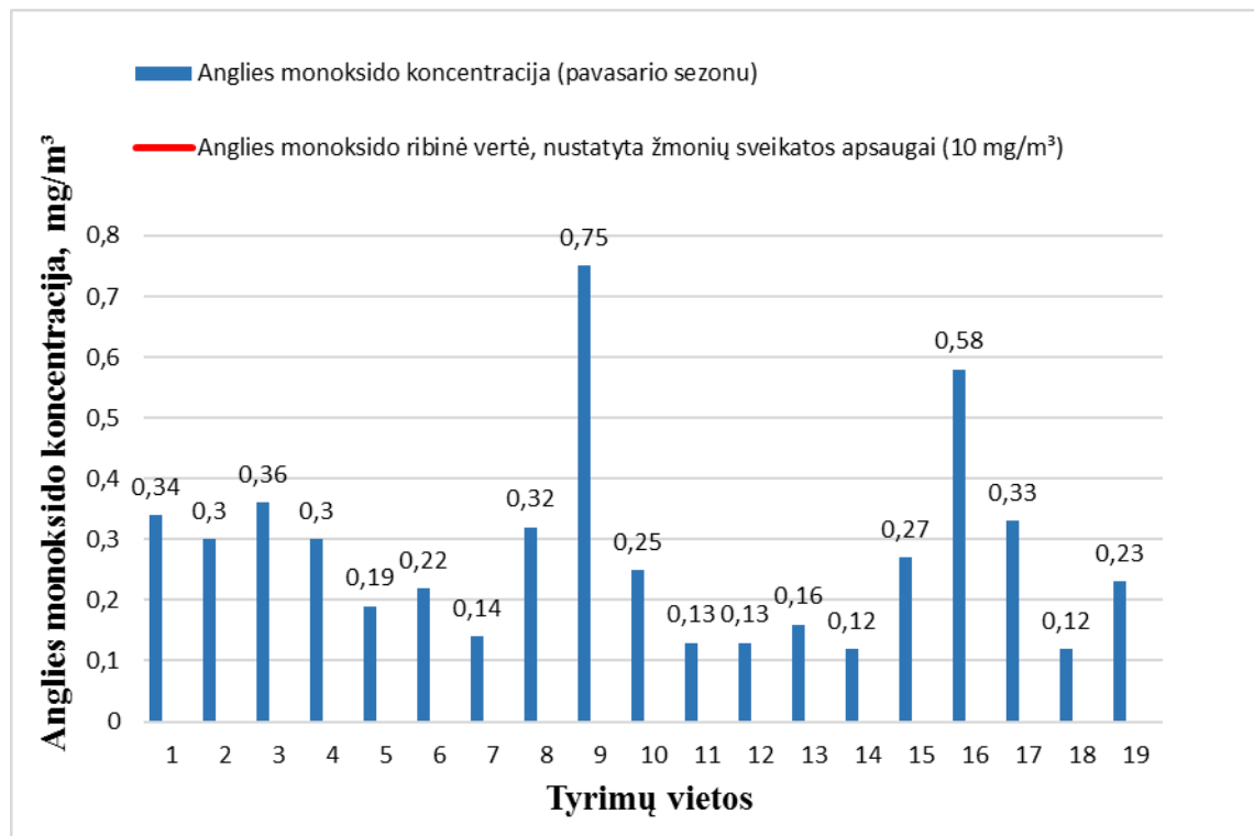
2.8 pav. Anglies monoksido (CO) koncentracija aplinkos ore Klaipėdos rajone 2020 m. pavasario sezono metu bei ribinė vertė, nustatyta žmonių sveikatos apsaugai ( 10 \text{ mg/m}^3 )
