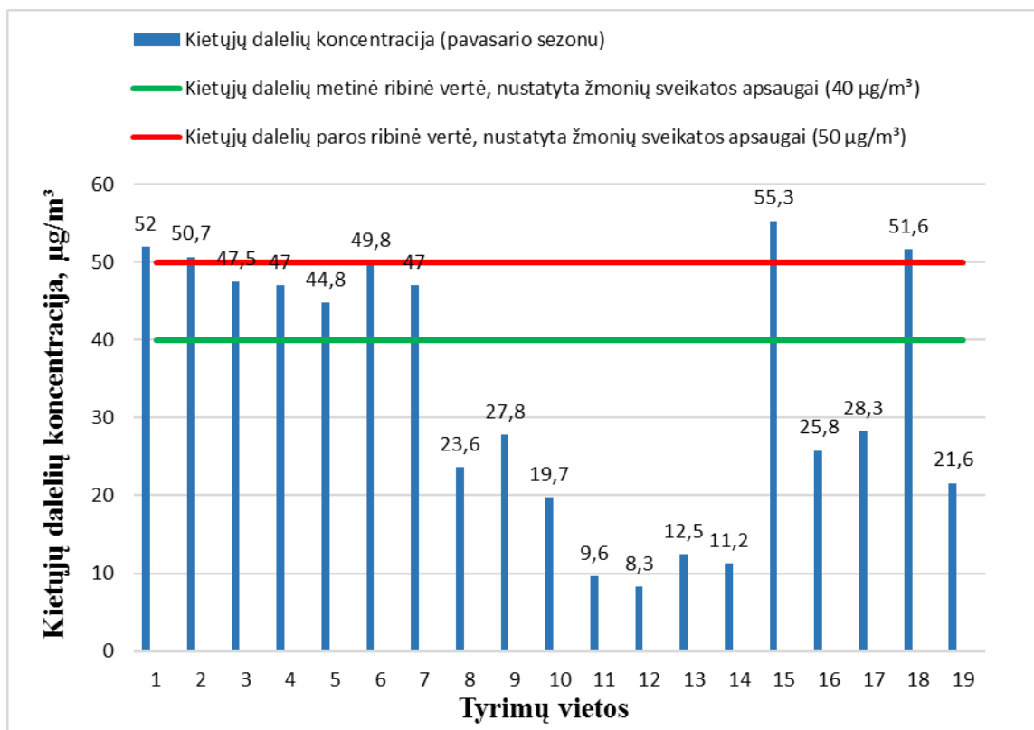
2.7 pav. Kietųjų dalelių (KD 10 ) koncentracija aplinkos ore Klaipėdos rajone 2020 m. pavasario sezono metu bei paros ribinė vertė, nustatyta žmonių sveikatos apsaugai (50 µg/m 3 ) ir metinė ribinė vertė, nustatyta žmonių sveikatos apsaugai (40 µg/m 3 )
