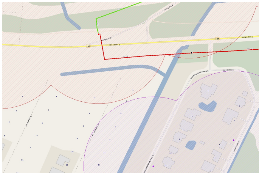
1 pav. Klaipėdos miesto ir rajono hidrantų išdėstymas.
