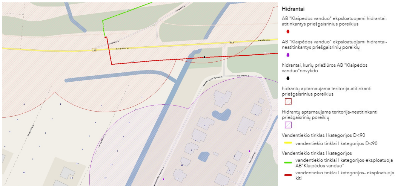
1 pav. Klaipėdos miesto ir rajono hidrantų išdėstymas.
