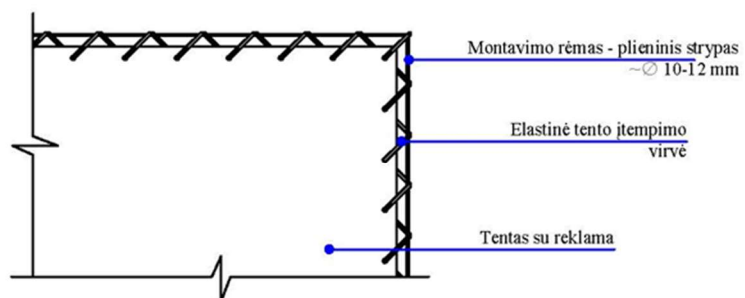
TENTO MONTAVIMO PRINCIPINĖ SCHEMA
