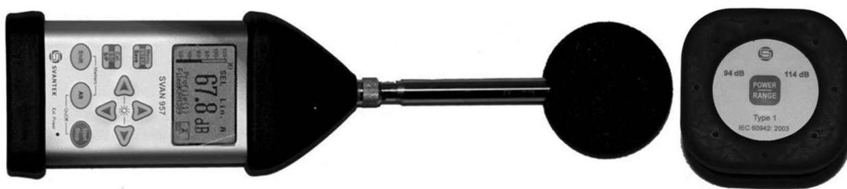
2 pav. SVAN 957 Triukšmo ir vibracijos matuoklis.
