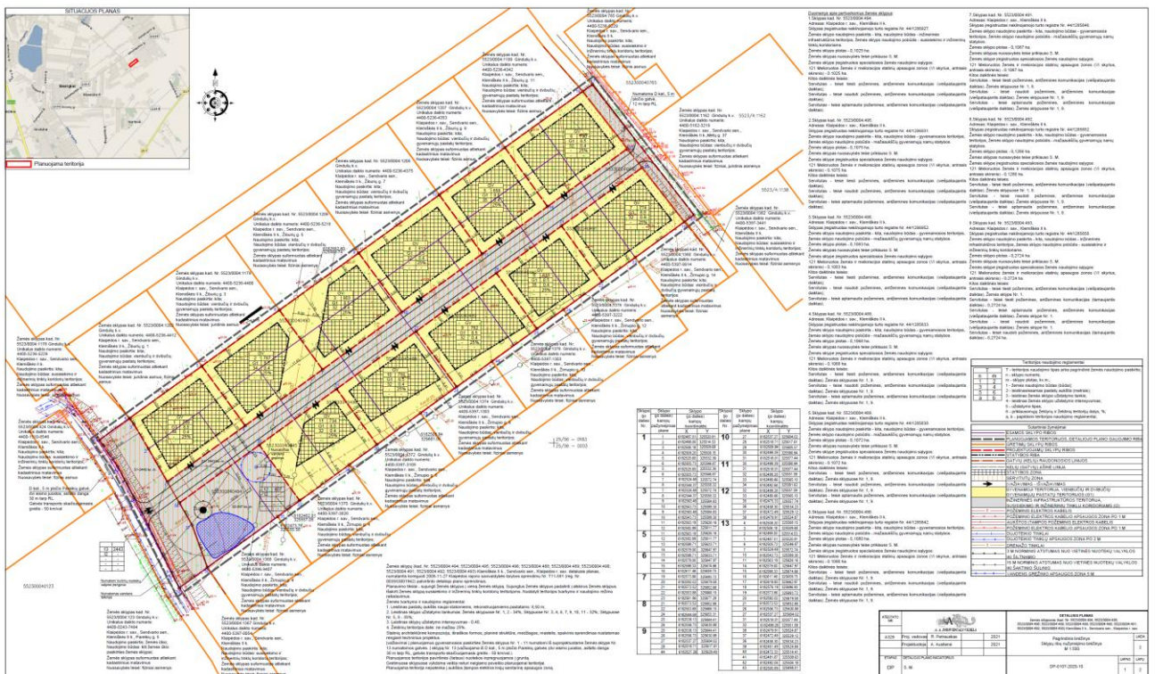
2 pav. Detalaus plano sprendiniai (planas mastelyje pateiktas prieduose).
